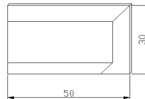
Pièce finition
