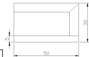
Pièce finition
